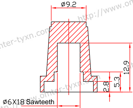
SEC.A-A
